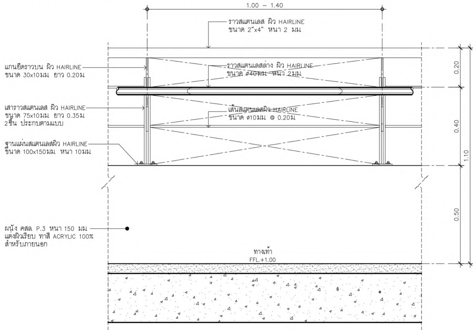
รูปด้านภายนอก แบบขยายรวางกันตง มาตราส่วน 1: 10
