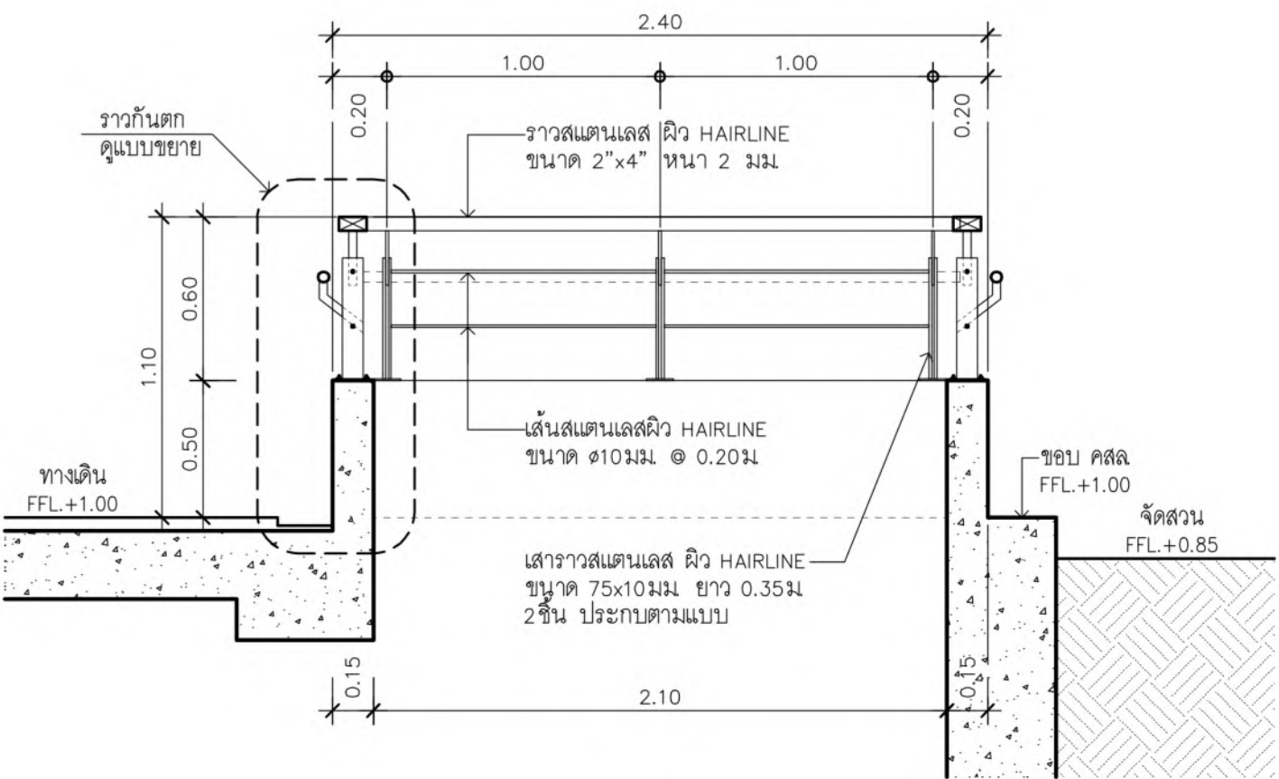
รูปตัด มาตราส่วน 1: 25
