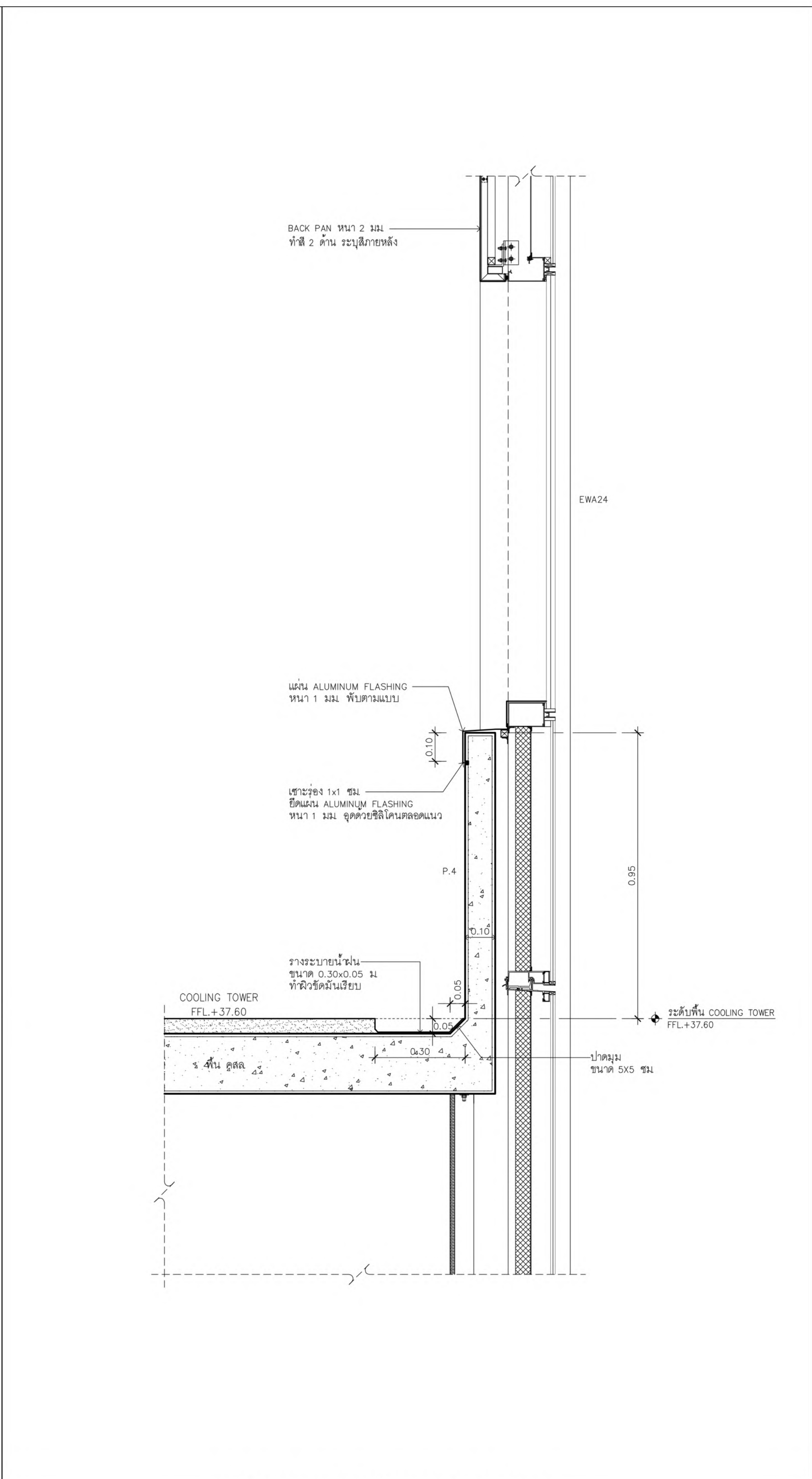
แบบขยาย รวากันตกภายนอก 6 มาตราส่วน 1:10
