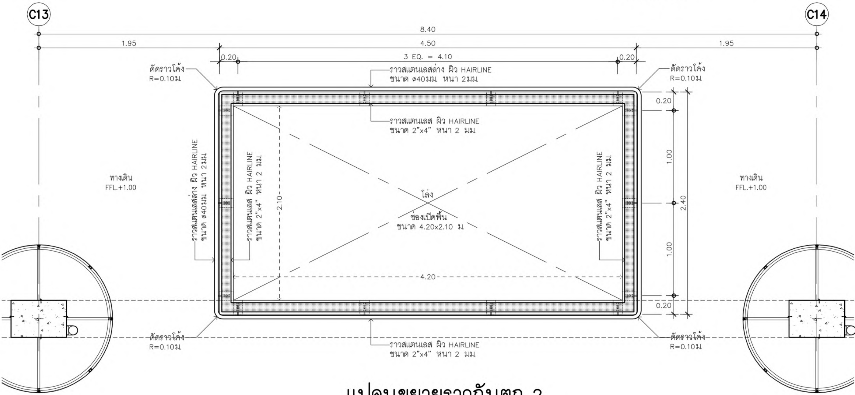
แปลนขยายรวางกันตง 2 มาตราส่วน 1: 25
