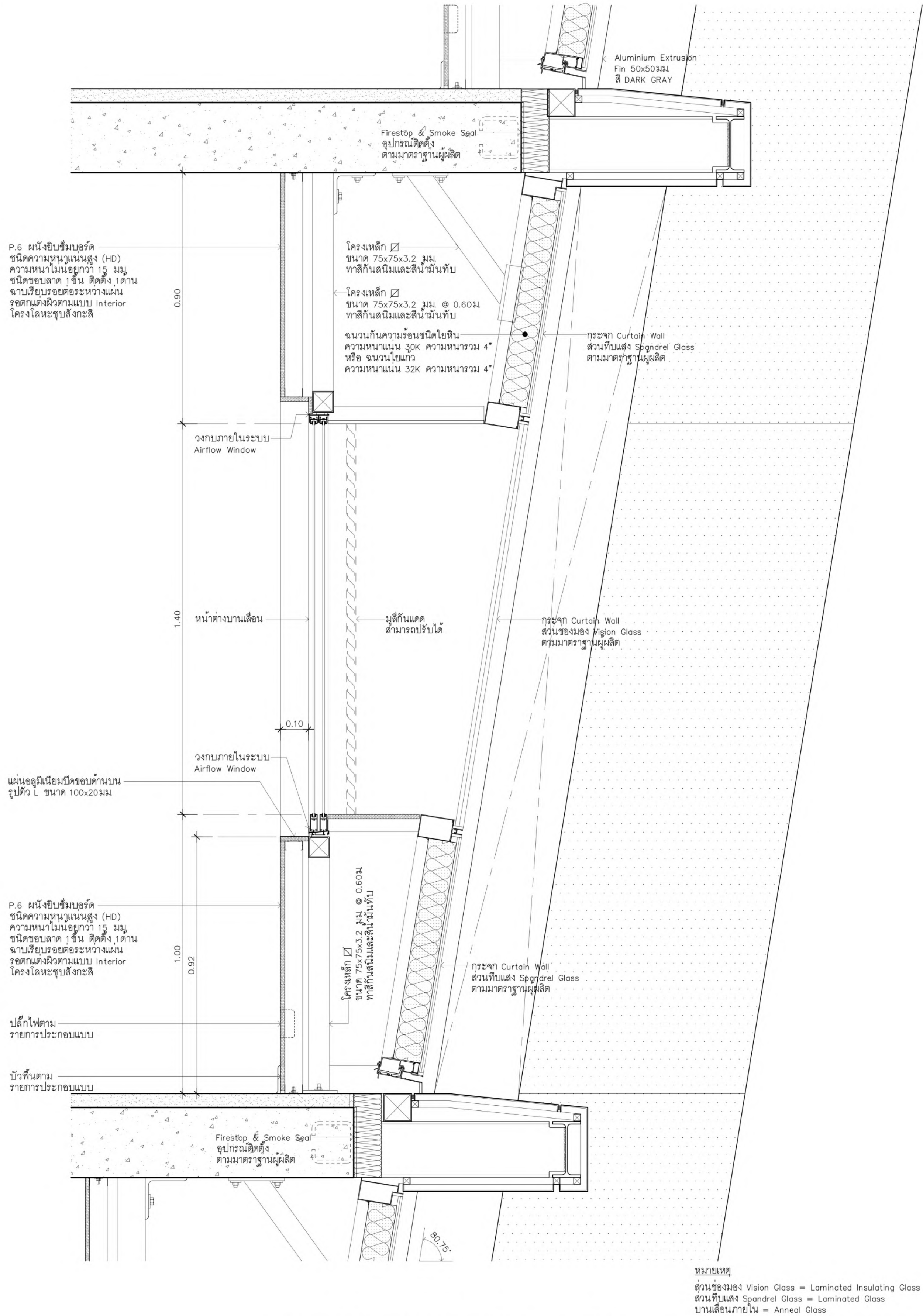
แบบขยายผนัง CURTAIN WALL 5 มาตราส่วน 1:10
