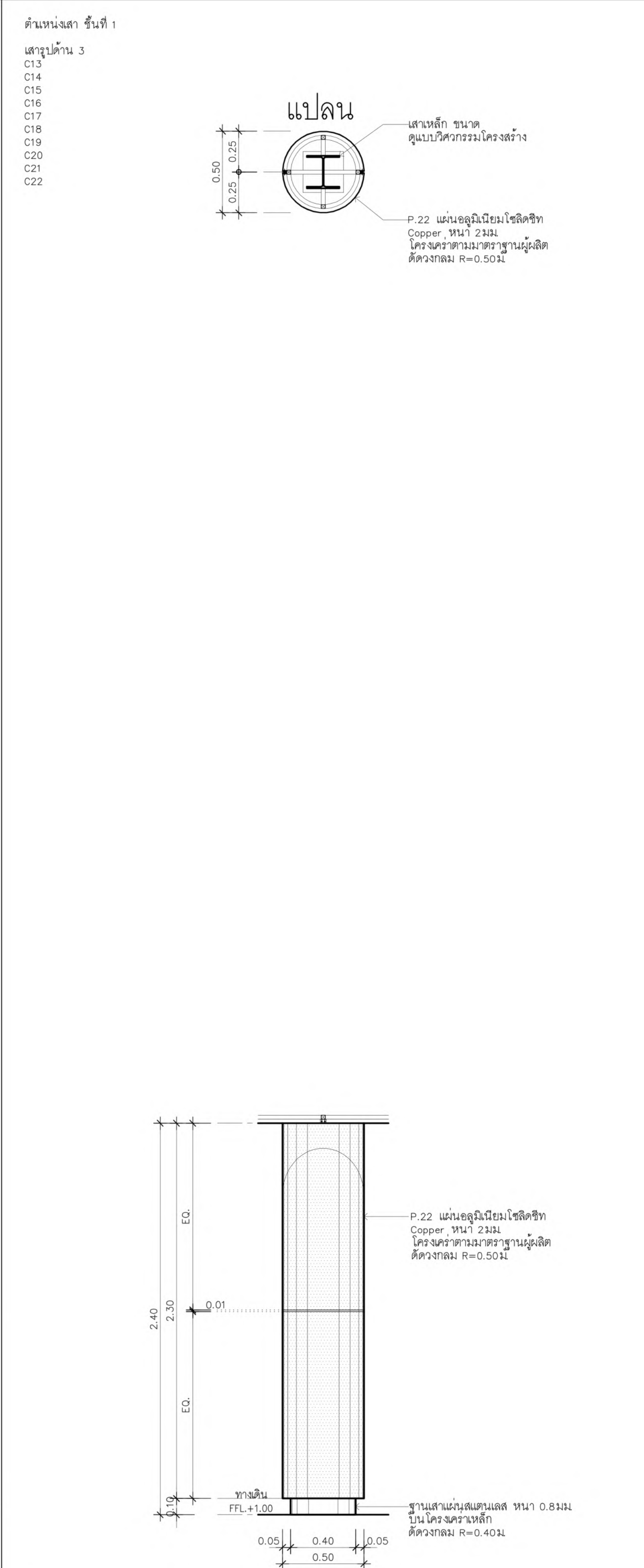
แบบขยาย เสาตกแต่งภายนอก 4 มาตราส่วน 1:20
