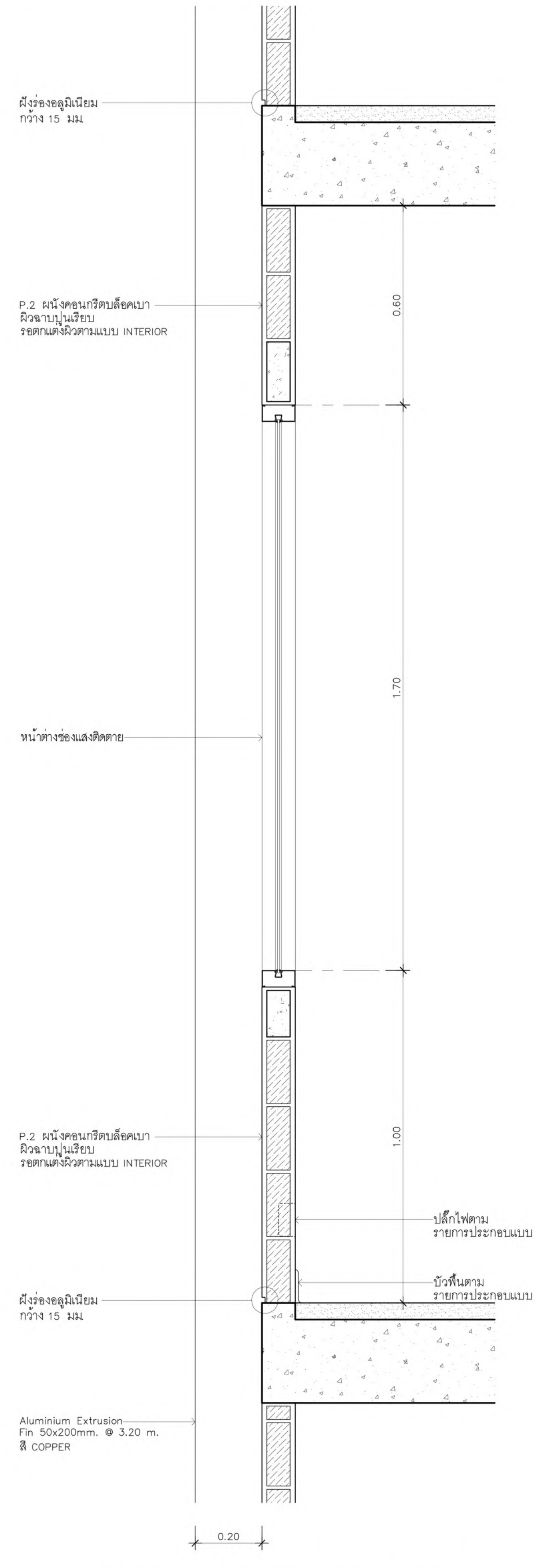
แบบขยายผนัง CURTAIN WALL 6 มาตราส่วน 1:10
