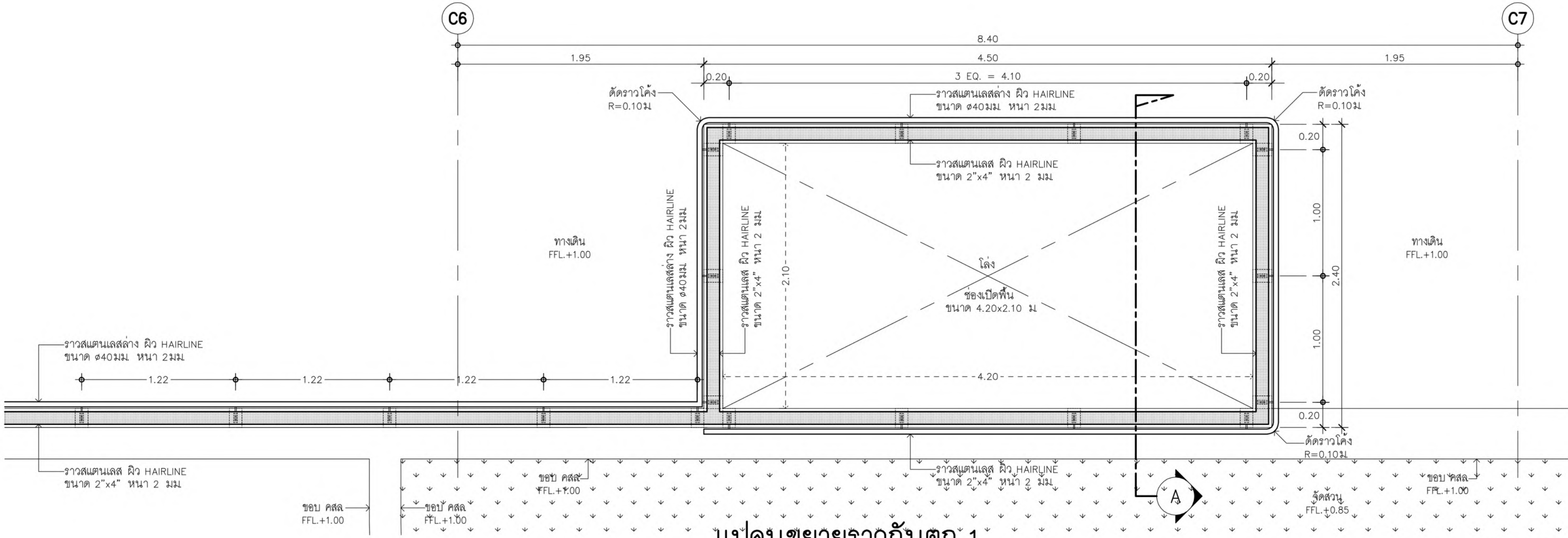
แปลนขยายรวางกันตง 1 มาตราส่วน 1: 25
