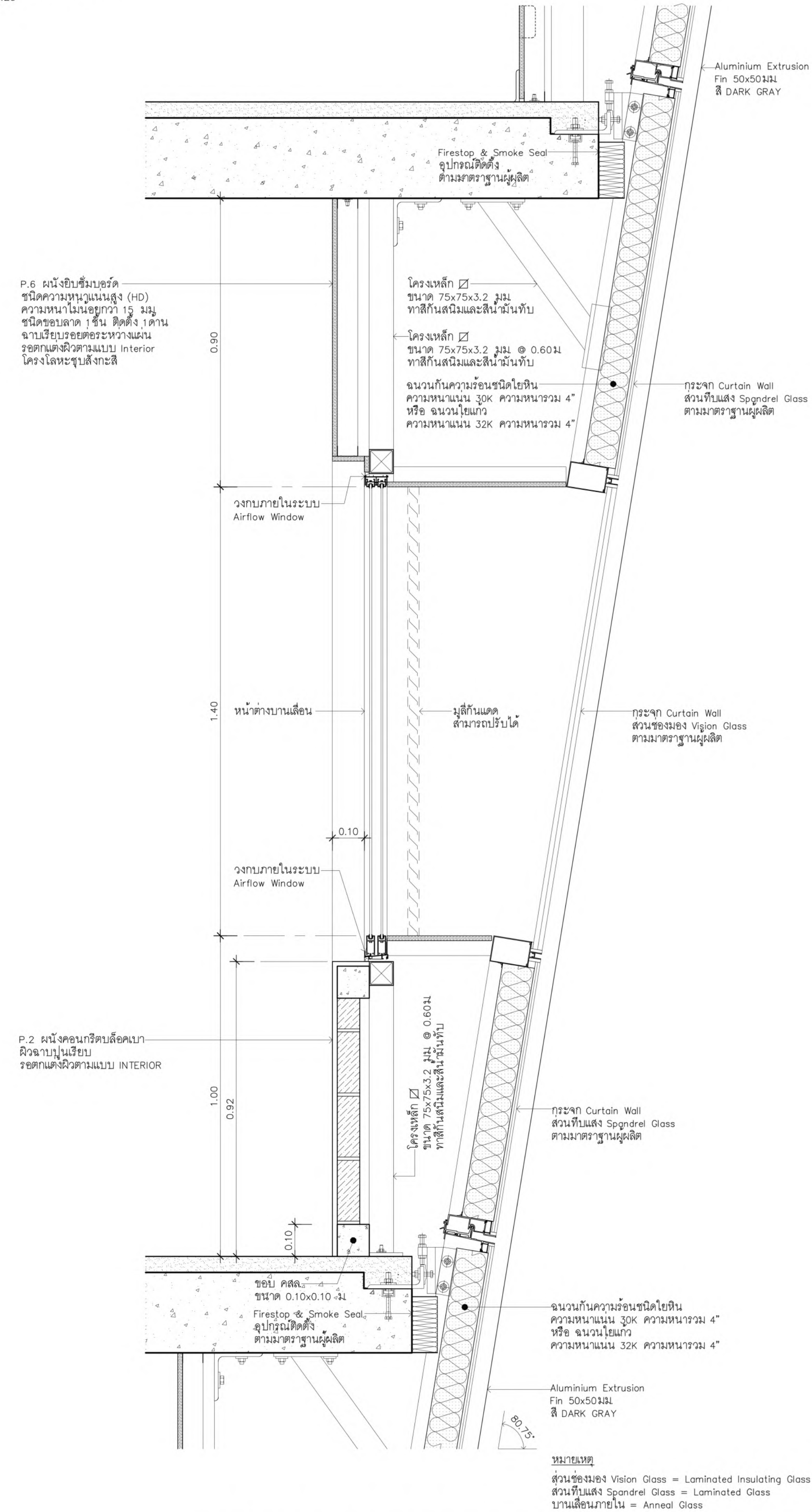
แบบขยายผนัง CURTAIN WALL 4.1 มาตราส่วน 1:10
